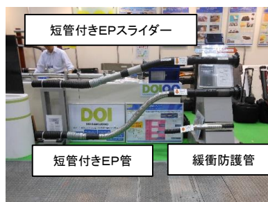
短管付きEPスライダー 短管付きEP管 緩衝防護管 公共建築設備工事標準図 仕様 耐震管路材「緩衝防護管 他」
