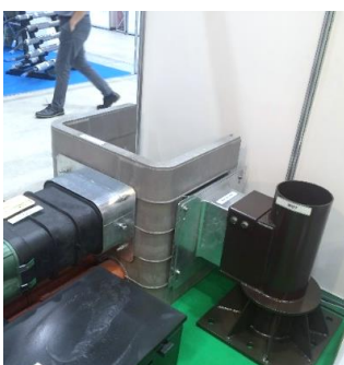
樹脂製品による軽量化 ※狭隘道路向け電線共同溝 鋼管柱(ソフト地中化)
