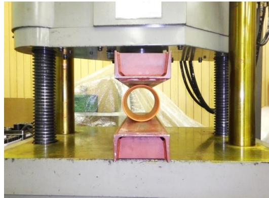
50t 万能試験装置（引張・圧縮）
