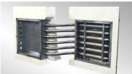
●自在伸縮継手(スプリング式)
